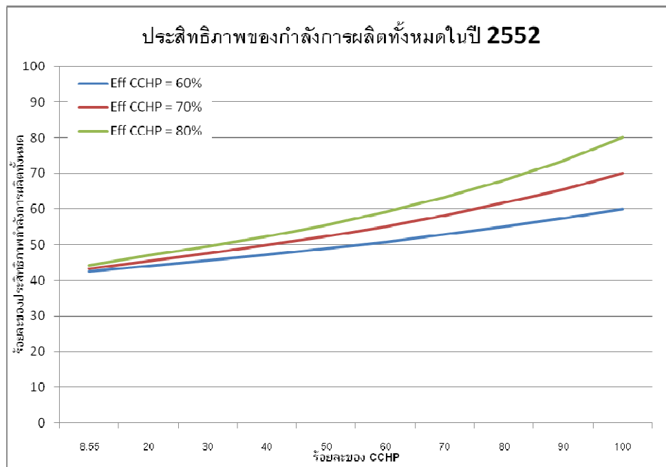
รูปที่ 4 ประมาณการประสิทธิภาพการใช้พลังงานปฏิกิริยาโดยรวมของโรงไฟฟ้าพลังความร้อนของประเทศไทย ในปี พ.ศ. 2552 หากปรับสัดส่วนกำลังผลิต CCHP เพิ่มขึ้นจนถึงร้อยละ 100
