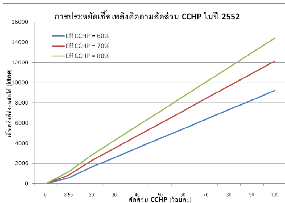
รูปที่ 5 ประมาณการปริมาณเชื้อเพลิงปฏิกิริยาที่สามารถประหยัดได้ ในหน่วย ktoe อ้างอิงข้อมูลปี พ.ศ. 2552 (สถานะปัจจุบัน) หากปรับสัดส่วนกำลังผลิต CCHP เพิ่มขึ้นจนถึงร้อยละ 100
